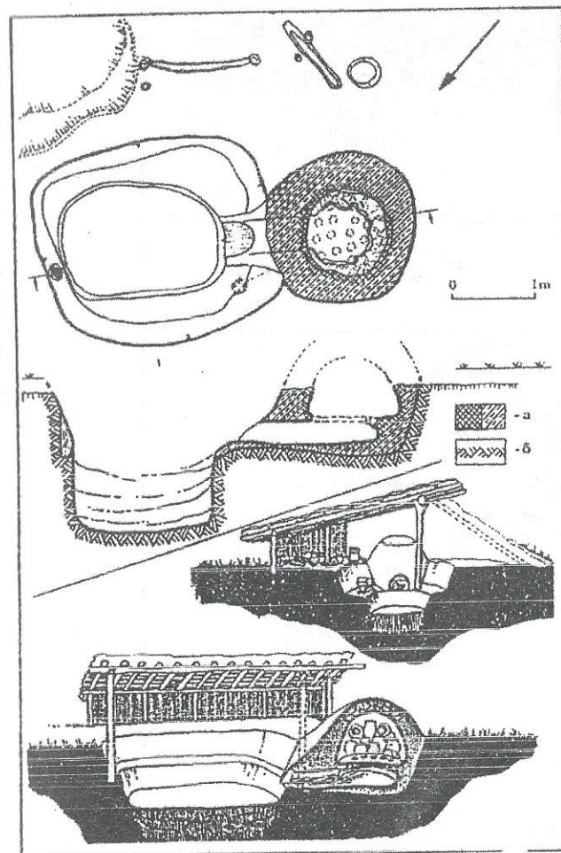
Рис. 2 – Горно № 6 з Автуничів (план, профіль (а – пропечена і обпалена глина, б – материк), зовнішній вигляд (реконструкція автора, Т.Г. Новик та П.Л. Корнієнка).
